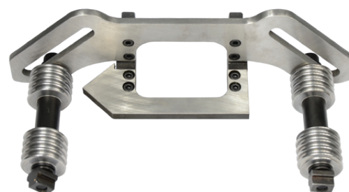
Piastra di guida standard universale in acciaio inox per la smussatura di lamiere e tubi con Ø 150-300mm (6-12")
