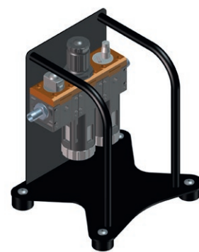
Filtere Régulateur Lubrificateur ZSP-0490-07-00-00
