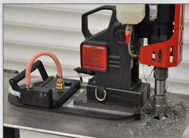
ALIMENTAZIONE ARIA COMPRESSA (configurazione opzionale)
