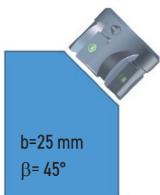
GLW-000056 Fräskopf
