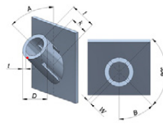
Tubo-piastra con fessure per staffe
