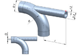
Connessione a gomito
