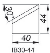
Cuțit de șanfrenare interioară la 30° Înălțime 44 mm [IB30/44] Cod produs: NOZ-000023
