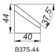
Cuțit de șanfrenare la 37,5° Înălțime 44 mm [B375/44] Cod produs: NOZ-000020
