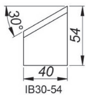
Cuțit de șanfrenare interioară la 30° Înălțime 54 mm [IB30/54] Cod produs: NOZ-000025
