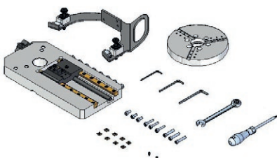
Accesorii pentru fațetare flanșă, inclusiv disc rotativ cu suport pentru trei cuțite de șanfrenare Cod produs: PRK-0807-06-00-00-0
