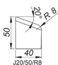
Cuțit de șanfrenare în J la 20°, Înălțime 50 mm, rază 8 mm [J20/50/R8] Cod produs: NOZ-000016
