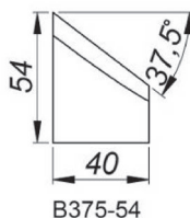
Cuțit de șanfrenare la 37,5° Înălțime 54 mm [B375/54] Cod produs: NOZ-000015
