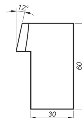
Cuțit de șanfrenare special la 12° Înălțime 60 mm Cod produs: NOZ-000086
