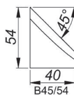
Cuțit de șanfrenare la 45° Înălțime 54 mm [B45/54] Cod produs: NOZ-000021
