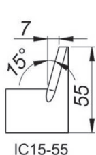
Cuțit de șanfrenare interioară la 15°, Înălțime 55 mm [IC15/55] Cod produs: NOZ-000001
