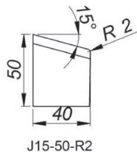
Cuțit de șanfrenare în J la 15° Înălțime 50 mm, rază 2 mm [J15/50/R2] Cod produs: NOZ-000022
