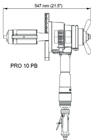
PRO-10 PB cu motor pneumatic
