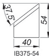
Cuțit de șanfrenare interioară la 37,5° Înălțime 54 mm [IB375/54] Cod produs: NOZ-000024
