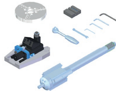
Set de accesorii ovale, inclusiv mandrină mare pentru țevă ID 0 126 - 296 mm (5 până la 11-5/8") și disc rotativ cu suport pentru trei cuțite de șanfrenare Cod produs: PRK-0807-07-00-00-0
