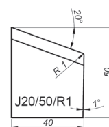
Cuțit de șanfrenare în J la 20°, Înălțime 50 mm, rază 1 mm [J20/50/R1] Cod produs: NOZ-000085
