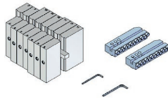
Set de extensie pentru OD până la 355 mm (14"), inclusiv 2 suporturi lungi de cuțite de șanfrenat și bacuri 7, 8, 9, 10, 11 Recomandat pentru grosimea peretelui țevilor de până la 7 mm (0,26") Cod produs: ZST-0807-08-00-00-0
