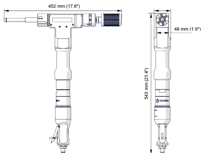
PRO 2 PB cu motor pneumatic
