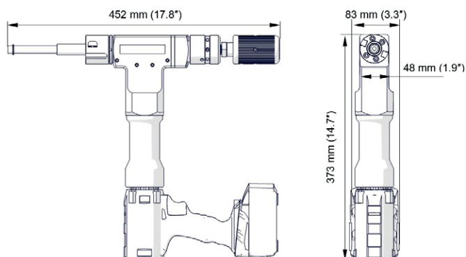
PRO 2 PB acționat cu baterii
